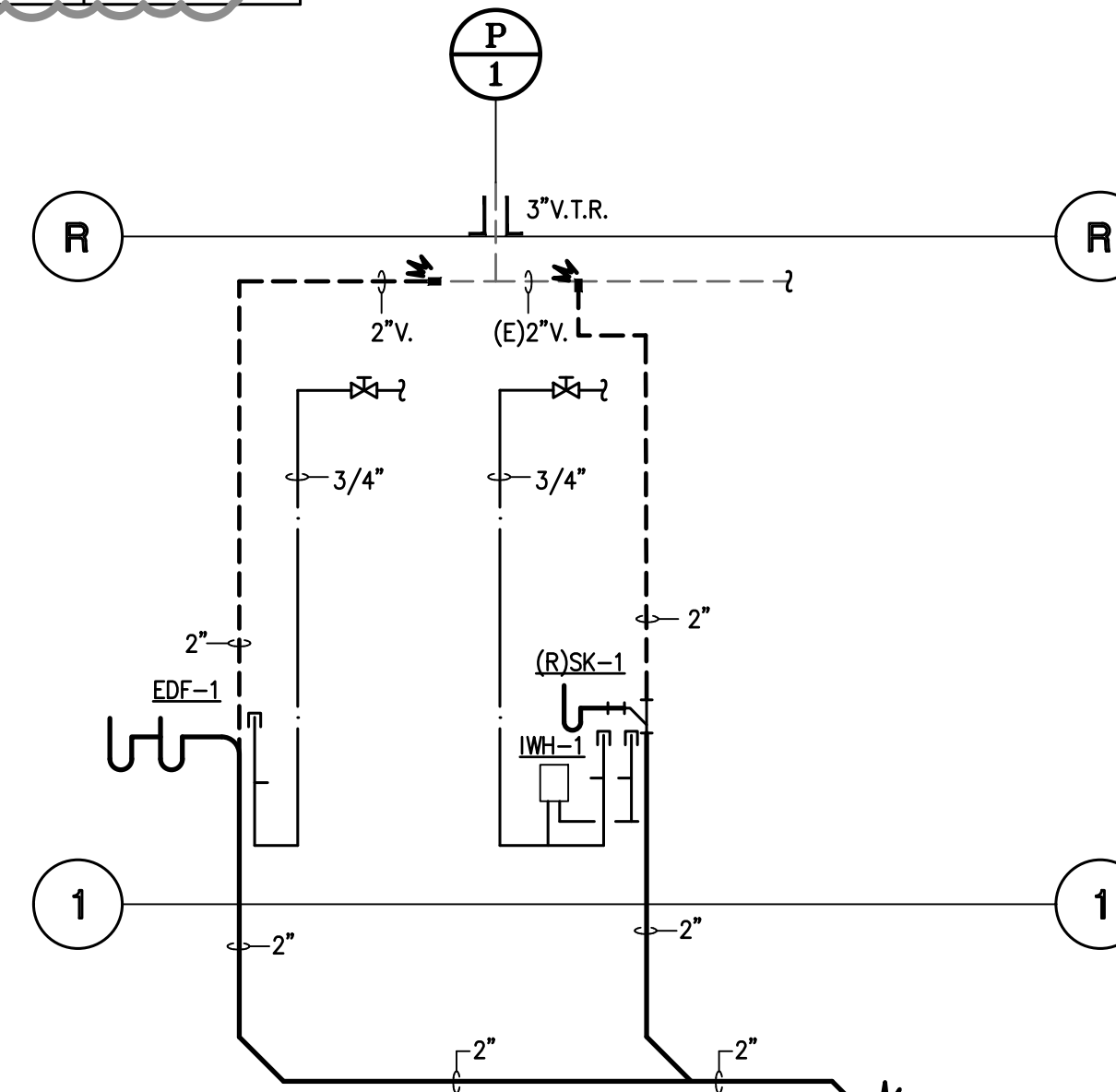
01 PLUMBING RISER DIAGRAM SCALE: NONE
